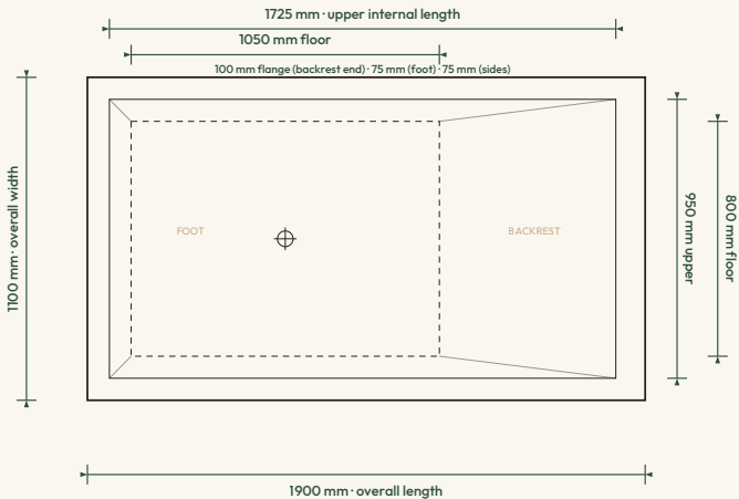
PLAN · BIRDSEYE
