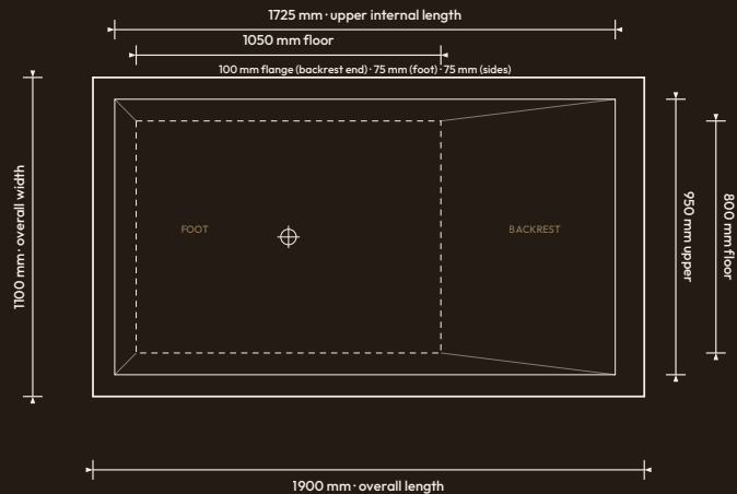
PLAN · BIRDSEYE
